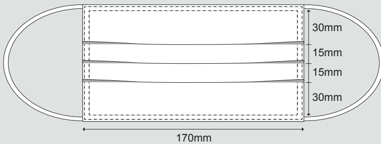
MÁSCARA DW-Mod.2 (sem ajuste metálico)
